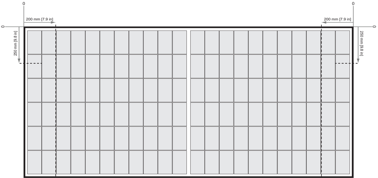
Fig. 10:Fijación de los paneles serie REC Alpha 72 con raíles cortos
