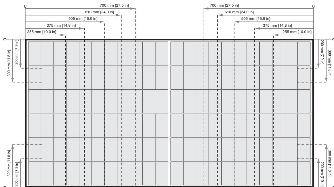
Fig. 8: Fijación de los paneles serie REC Alpha Pure con raíles cortos
