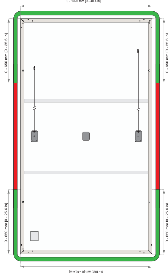
Fig. 24: Zonas de instalación de dispositivos MLPE en la serie REC Alpha 72
