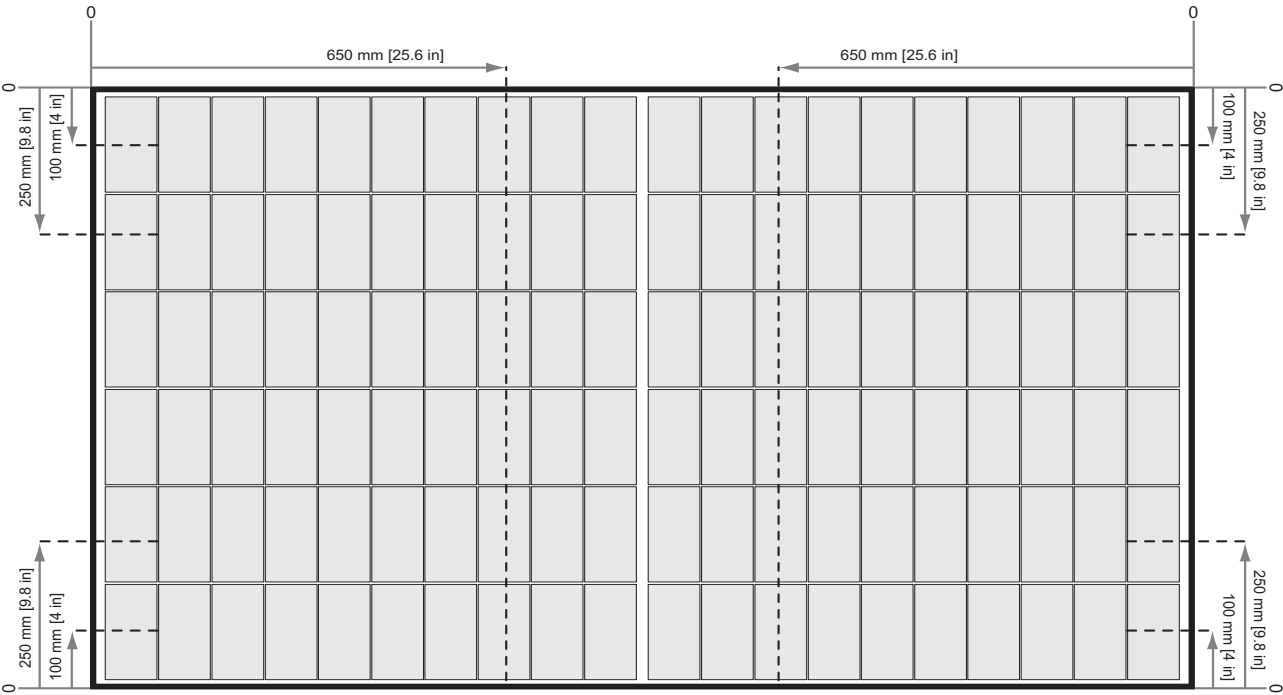
Fig. 4: Fijación de paneles serie REC Alpha con raíles paralelos al lado largo del panel
