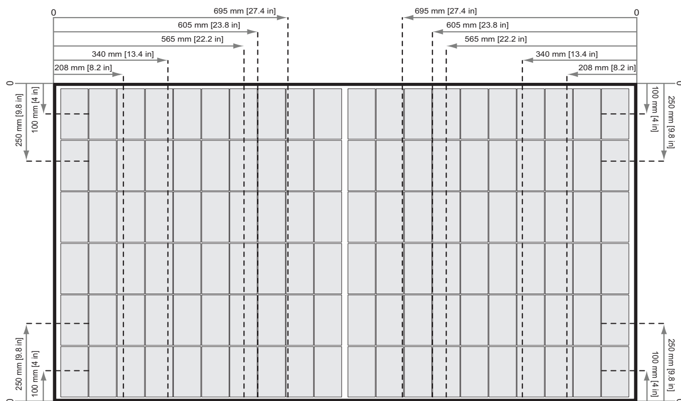
Fig. 3: Fijación de paneles serie REC Alpha con ralles paralelos al lado corto del panel
