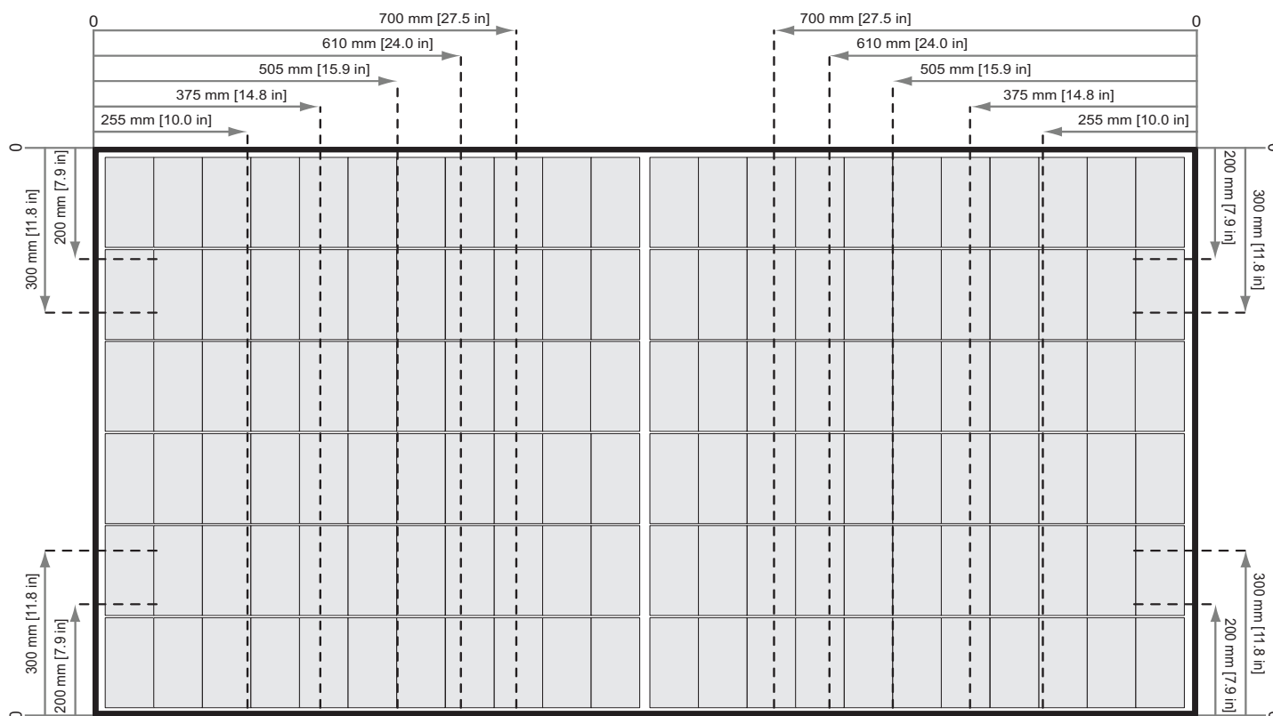
Fig. 6: Fijación de paneles serie REC Alpha Pure con ralles paralelos al lado corto del panel
