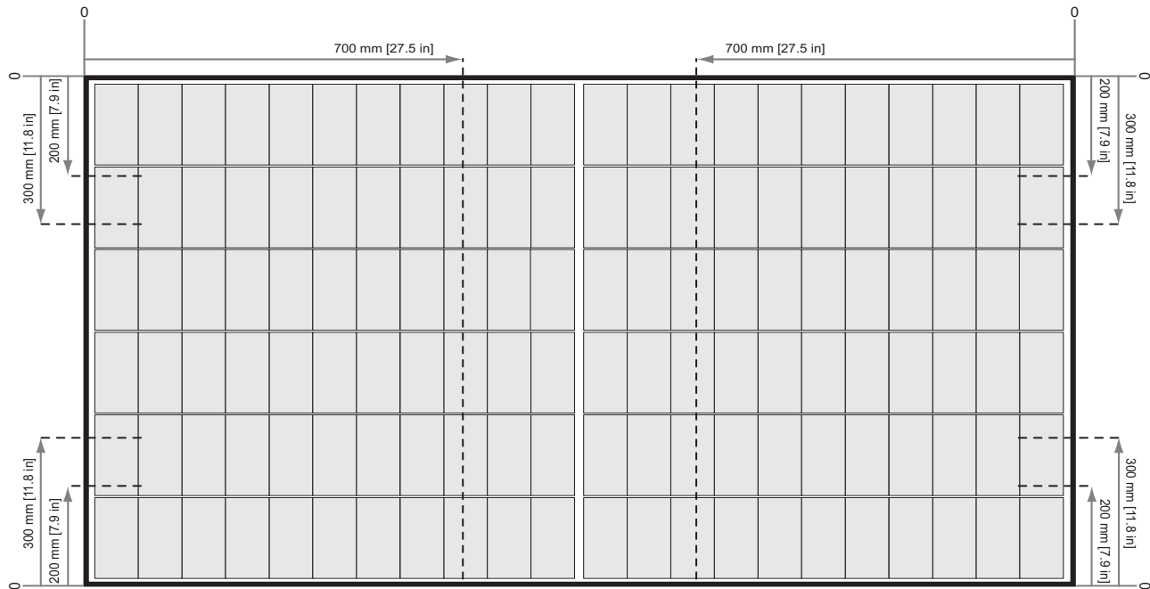
Fig. 7: Fijación de paneles serie REC Alpha Pure con ralles paralelos al lado largo del panel
