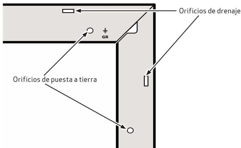
Fig. 15: Orificios de drenaje y puesta a tierra
