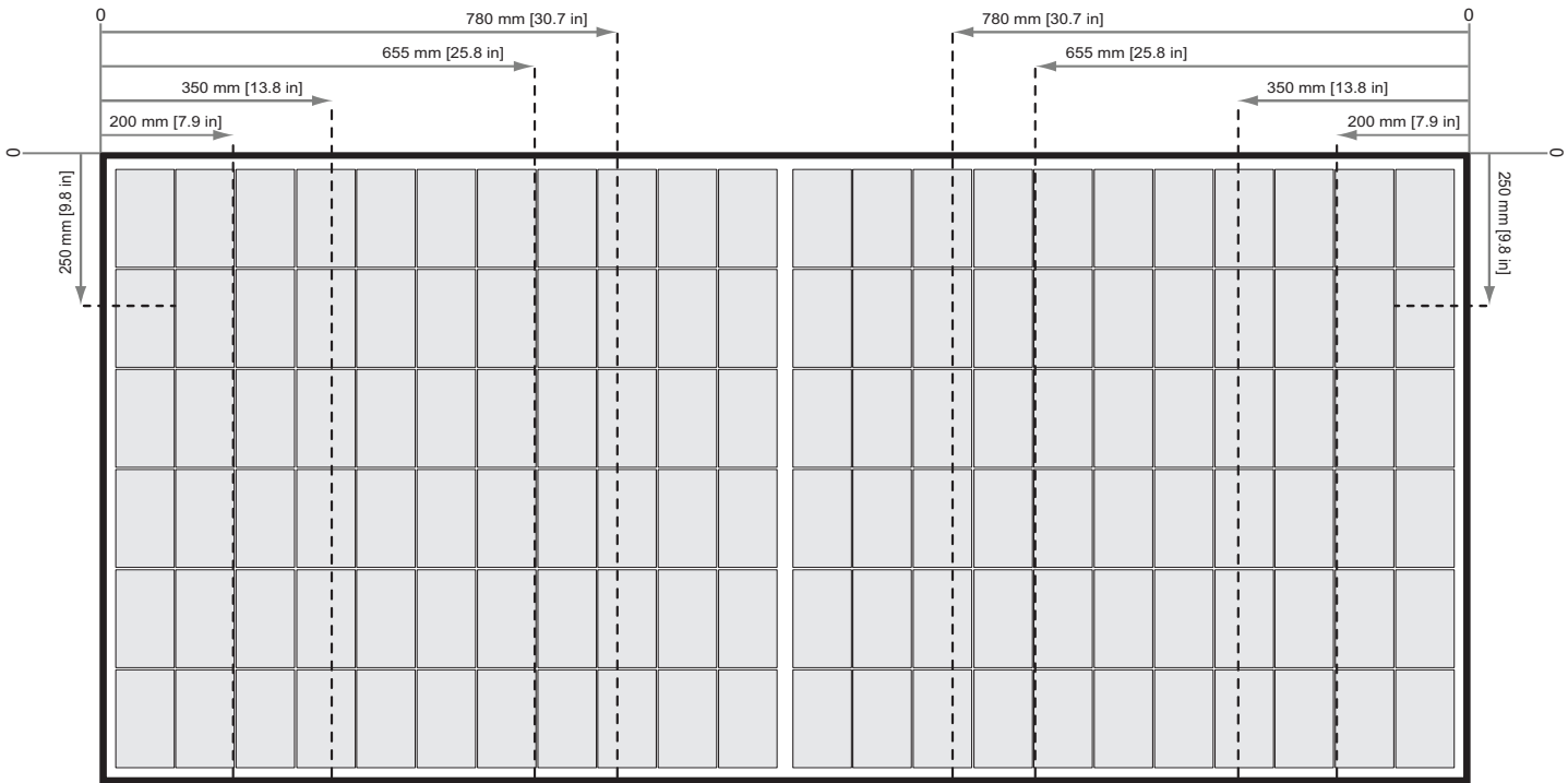
Fig. 9: Fijación de paneles serie REC Alpha 72 con ralles paralelos al lado corto del panel
