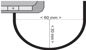
Fig. 17: Radio de flexión mínimo del cable
