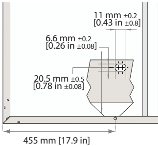
Fig. 11: Orificios de montaje: Serie REC Alpha
