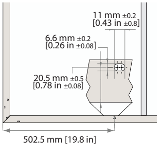
Fig. 12: Orificios de montaje: Serie REC Alpha 72
