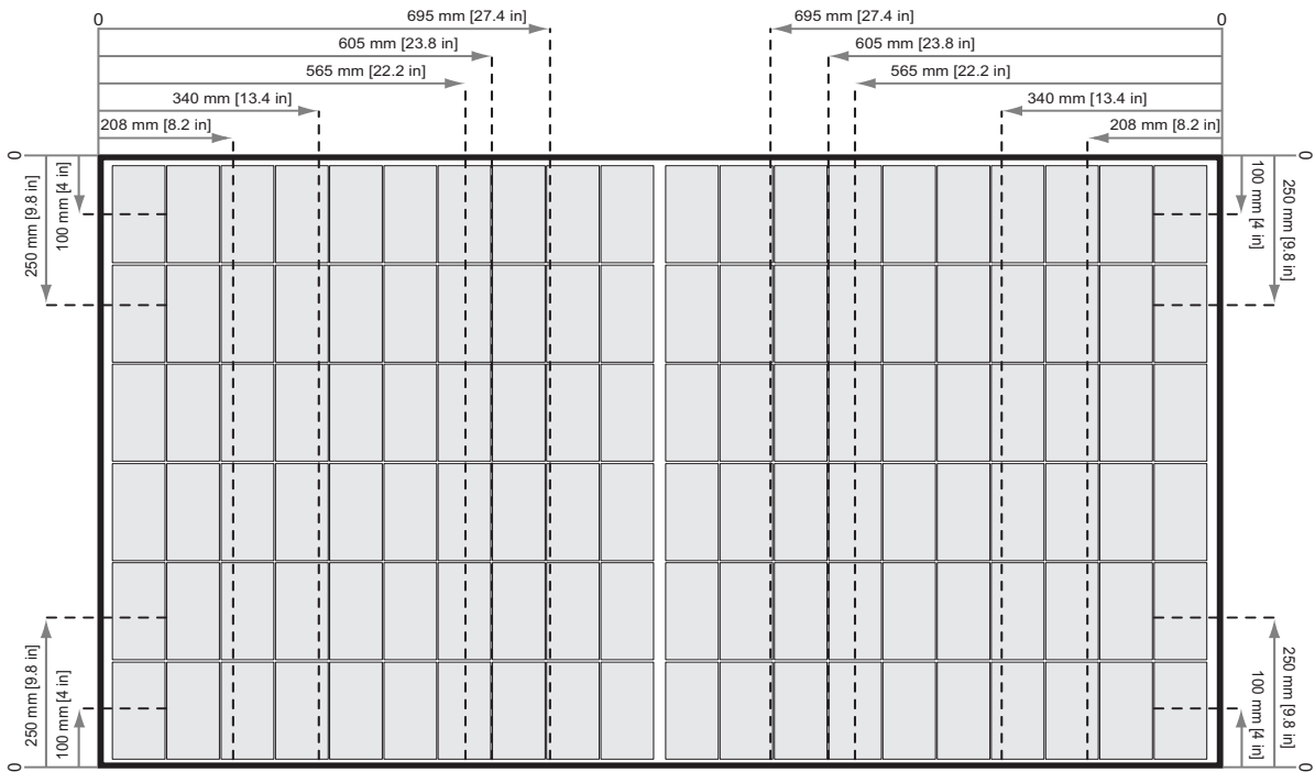
Fig. 5: Fijación de los paneles serie REC Alpha con ralles cortos
